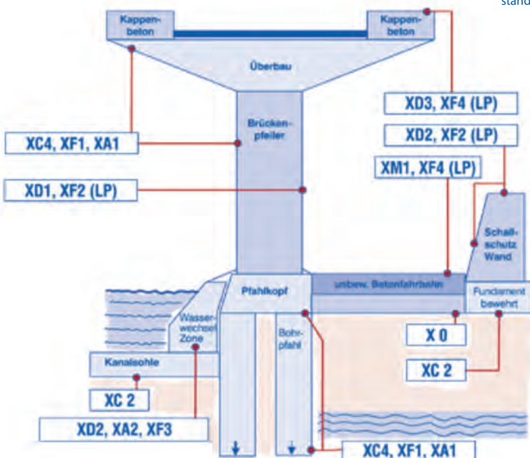
Beispiele für Beton im Ingenieurbau. Für die richtige Auswahl der Betonsorte, ist allein der Abnehmer verantwortlich.
