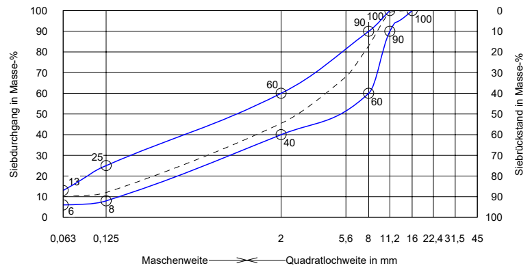
Sieblinienbereich für AC 11 TD*
